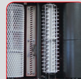
Gitterwalzen, Igelwalze, Glattwalze, Saatgutauslauf
