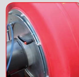
Stufenlose Turbinenverstellung über Drehhebelverschluss
