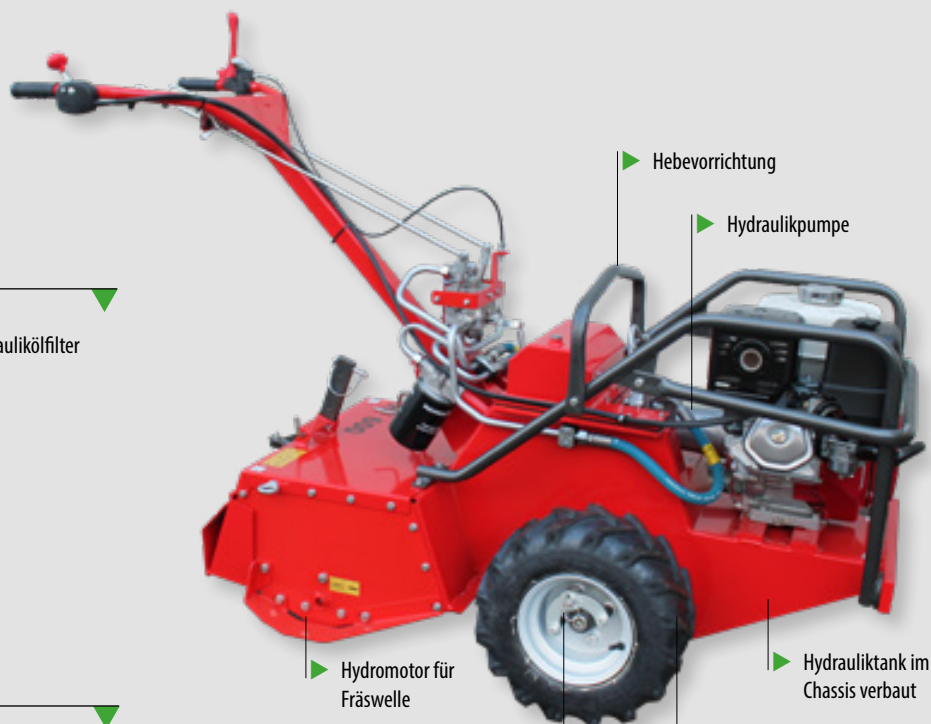
Hydrostatischer Fahrtrieb
