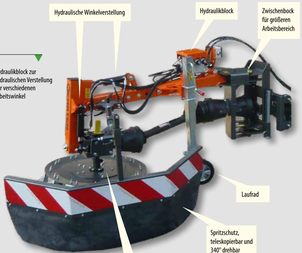
Getriebe drehbar für beide Laufrichtungen
